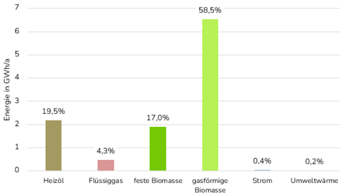
Abbildung 18: Wärmeverbrauch nach Energieträger (Veröffentlichung nach WPG, Anlage 2, I.)
