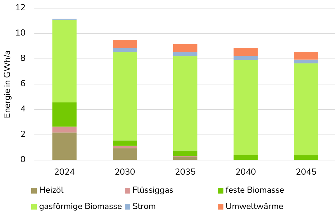
Abbildung 49: Wärmeverbrauch nach Energieträger in den Stützjahren (Veröffentlichung nach WPG, Anlage 2, III.)
