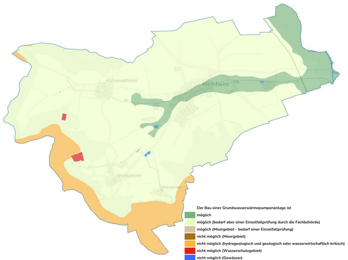
Abbildung 37: Potenziale für Grundwasserwärmepumpen (Veröffentlichung nach WPG, Anlage 2, II.) [Quelle: Bayerisches Landesamt für Umwelt, www.ifu.bayern.de ]
