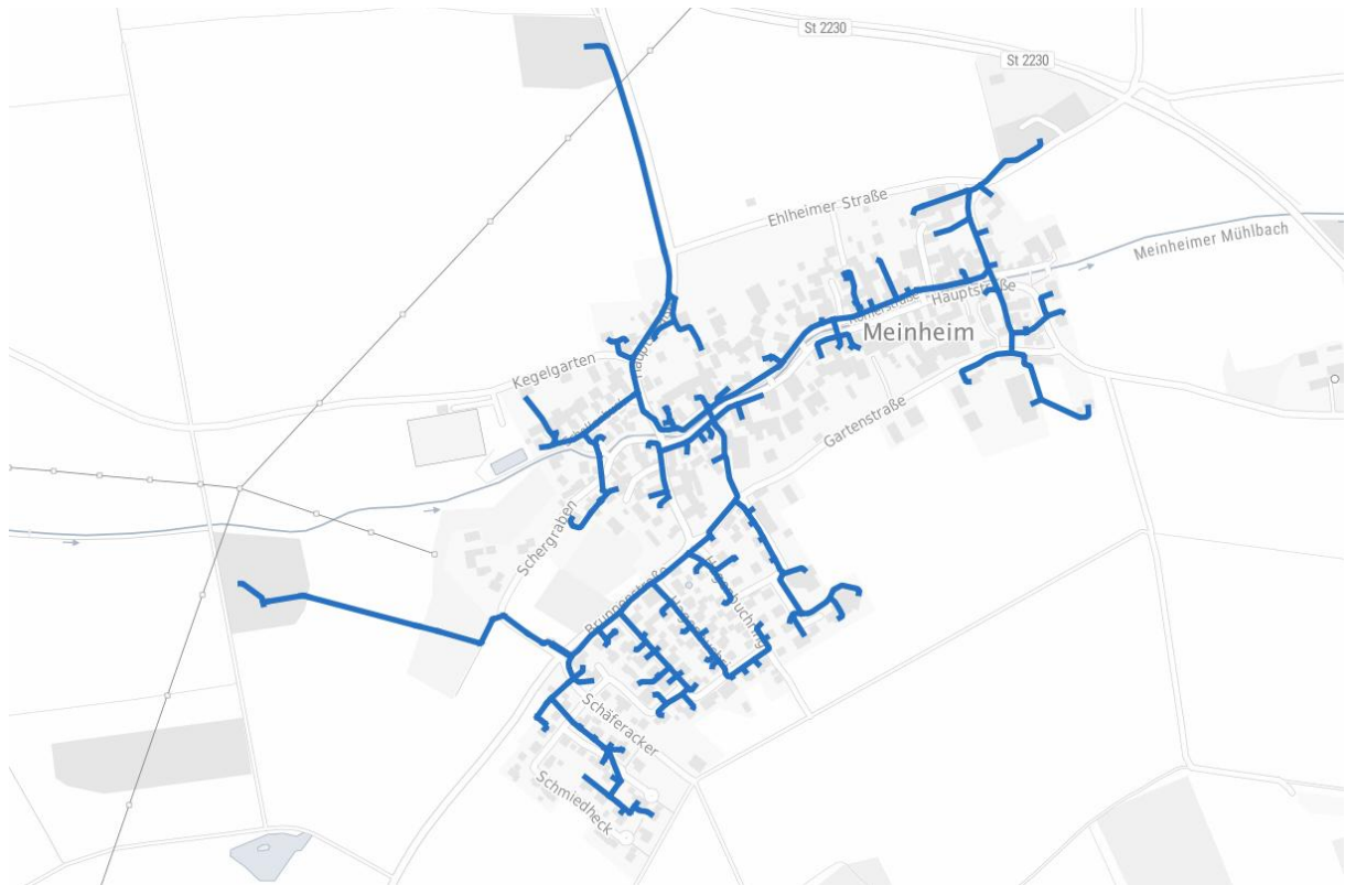
Abbildung 10: Wärmenetz Meinheim (Veröffentlichung nach WPG, Anlage 2, I.)
