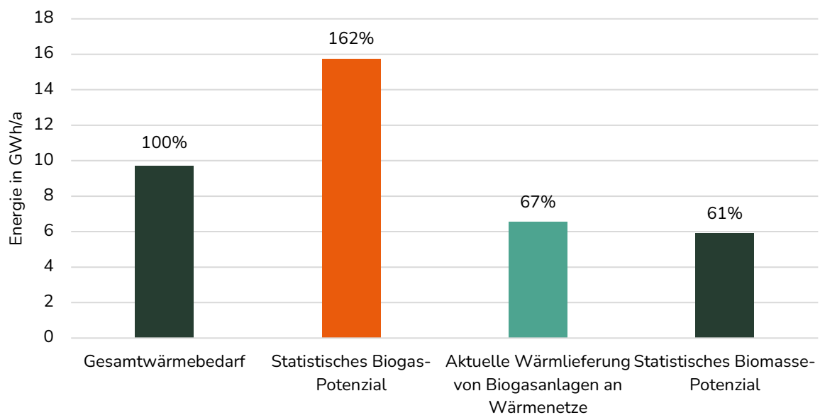
Abbildung 40: Gegenüberstellung Biogaspotenzial mit Gesamtwärmeverbrauch und bereits genutztem Biogas
