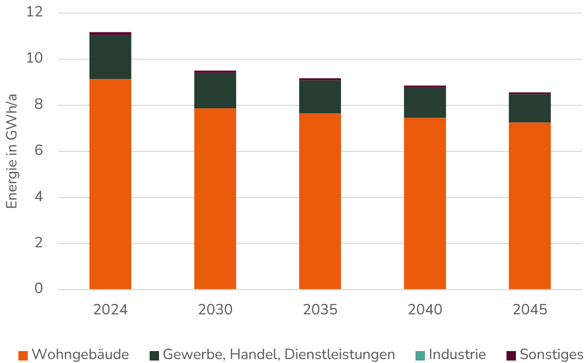
Abbildung 50: Endenergieverbrauch nach Sektoren in den Stützjahren (Veröffentlichung nach WPG, Anlage 2, III.)
