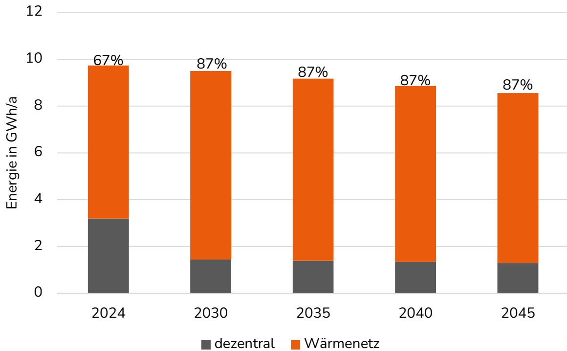
Abbildung 51: Anteil leitungsgebundener Wärme am gesamten Endenergieverbrauch in den Stützjahren (Veröffentlichung nach WPG, Anlage 2, III.)
