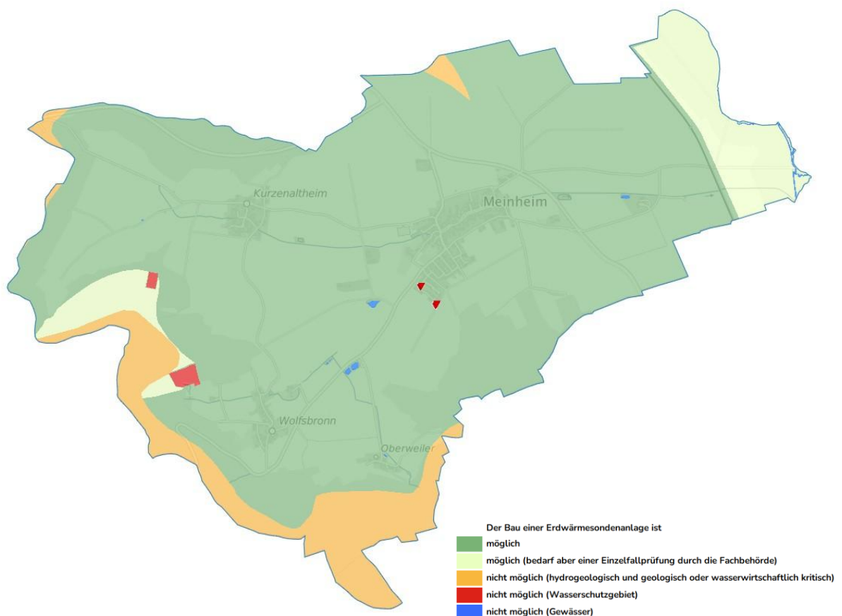
Abbildung 35: Potenziale für Erdwärmesonden (Veröffentlichung nach WPG, Anlage 2, II.) [Datenquelle: Bayerisches Landesamt für Umwelt, www.ifu.bayern.de ]
